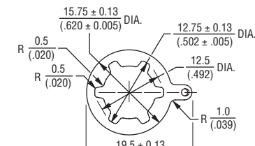
SOLDER LUG WASHER
