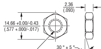
HEX NUT
