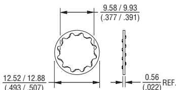
LOCKWASHER
