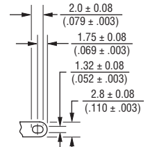
SOLDER LUG WASHER
